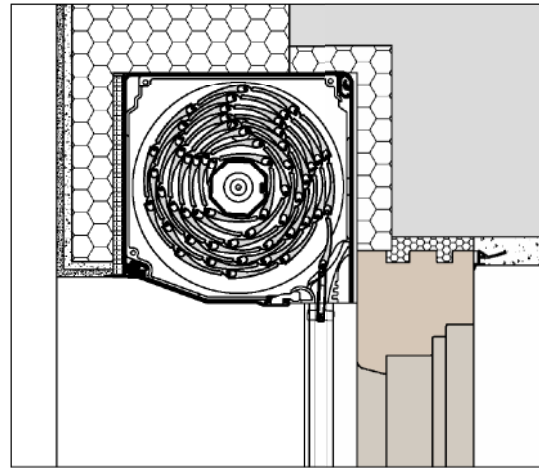
Sturzdämmung bauseits
